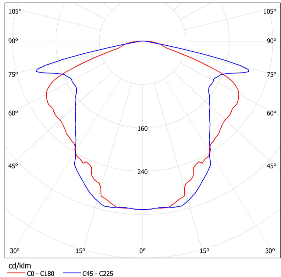
Кривая распределения сил света для светильника MIZAR LED
