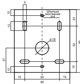
Монтажная пластина
