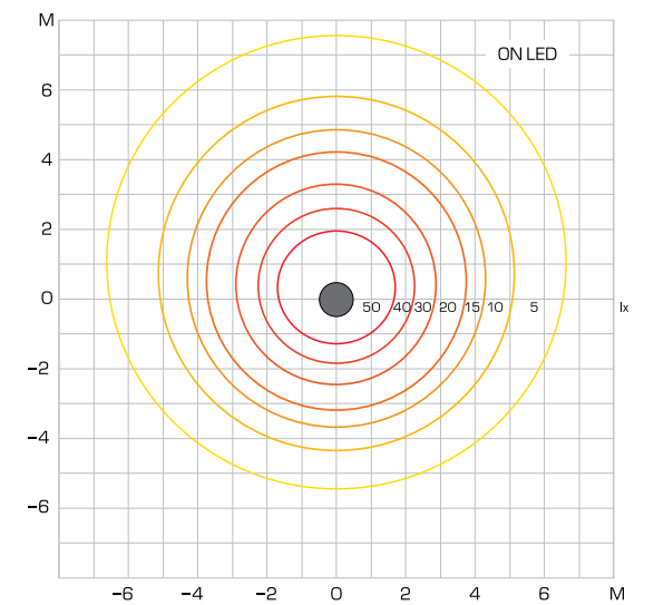
Диаграмма освещенности
