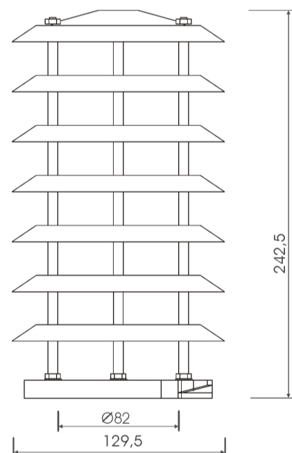
Растр большой вверх
