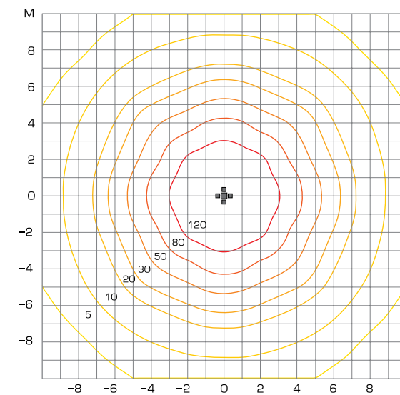
Диаграмма освещенности, lx
