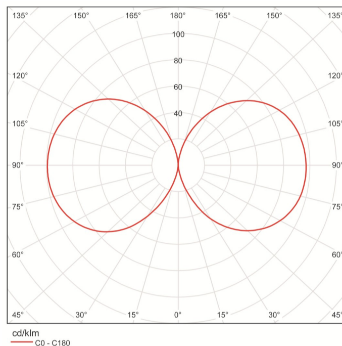
Кривая сил света SAL DECO-3 LED
